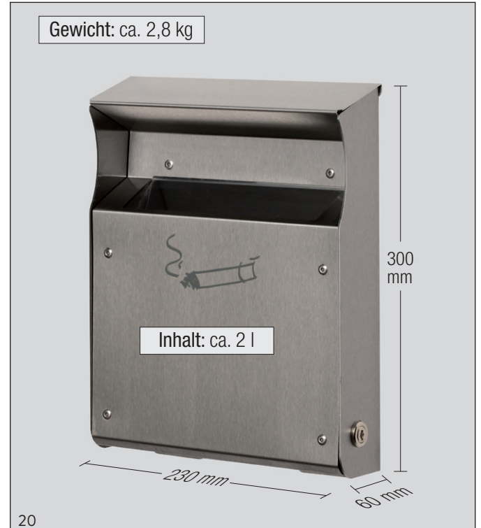
Abb.: Wandascher WH 28 Edelstahl, Art.-Nr. 45007
